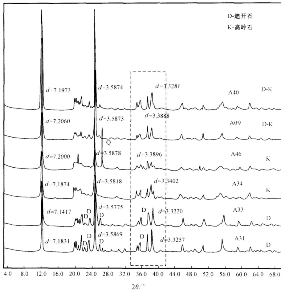
图 2 昌化田黄的粉晶 X 射线衍射图谱
