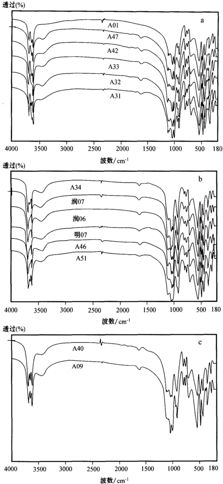
图 1 昌化田黄代表性样品的红外光谱图
