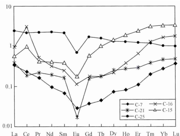
图5 样品的稀土元素配分模式图
