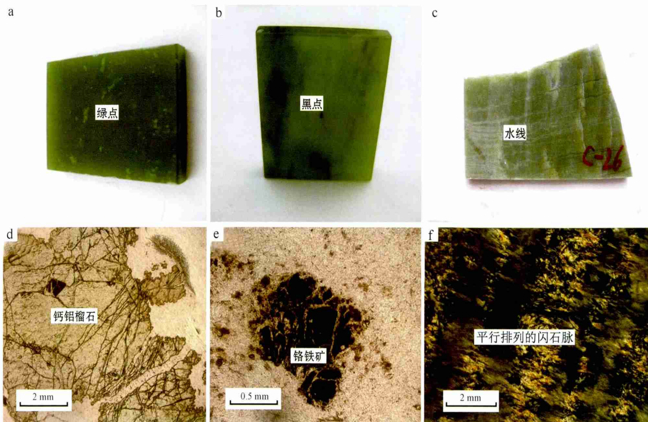
图 3 样品中的特殊结构
