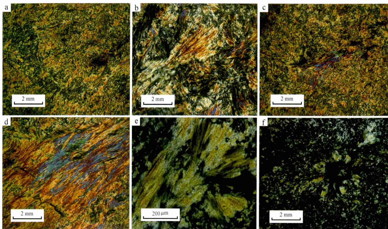
图 2 透闪石的显微结构(正交偏光)
